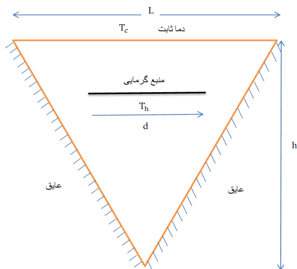
شکل ۲-۱- هندسه مورد بررسی در تحقیق کریمی و همکاران (منبع: ...)
